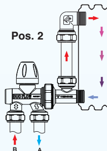
Collegamento con ingresso invertito Reversed inlet connection
