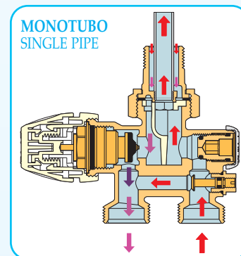
Collegamento con ingresso invertito Reversed inlet connection
