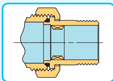
TENUTA CON O-RING O-RING
