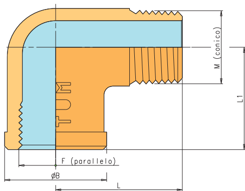
ART. 1561DIN raccordo curvo maschio/femmina serie pesante (DIN) ART. 1561DIN elbow male/female connector heavy model (DIN)
